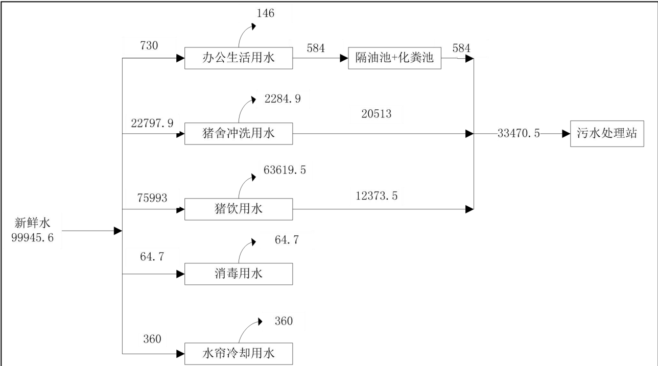
图 3-2-5 项目水平衡图 单位：m³/a
