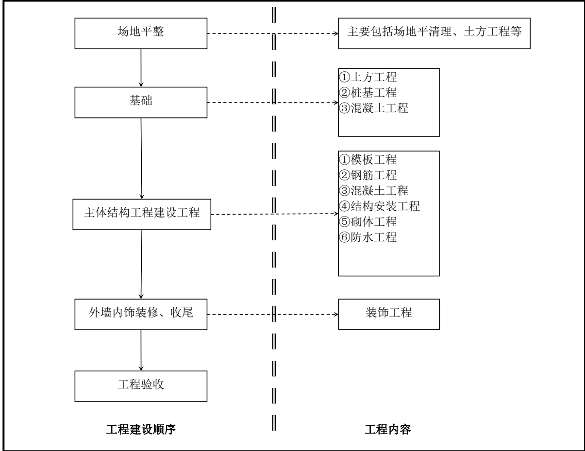
图 3-1-1 施工期总体工艺流程示意图
