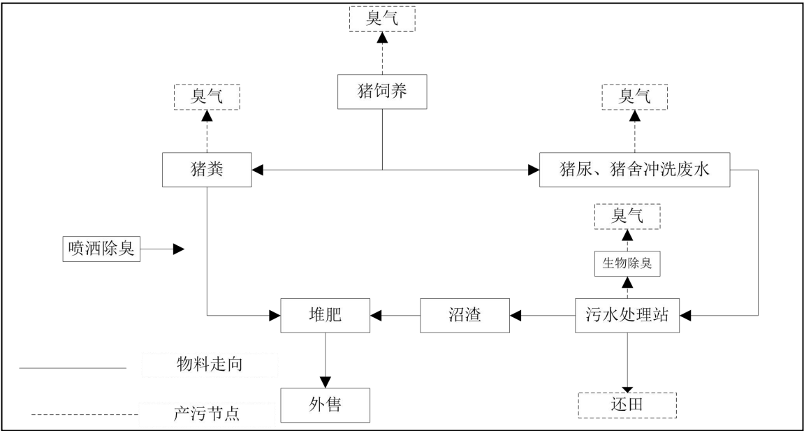
图 3-2-1 工艺流程及排污节点图
