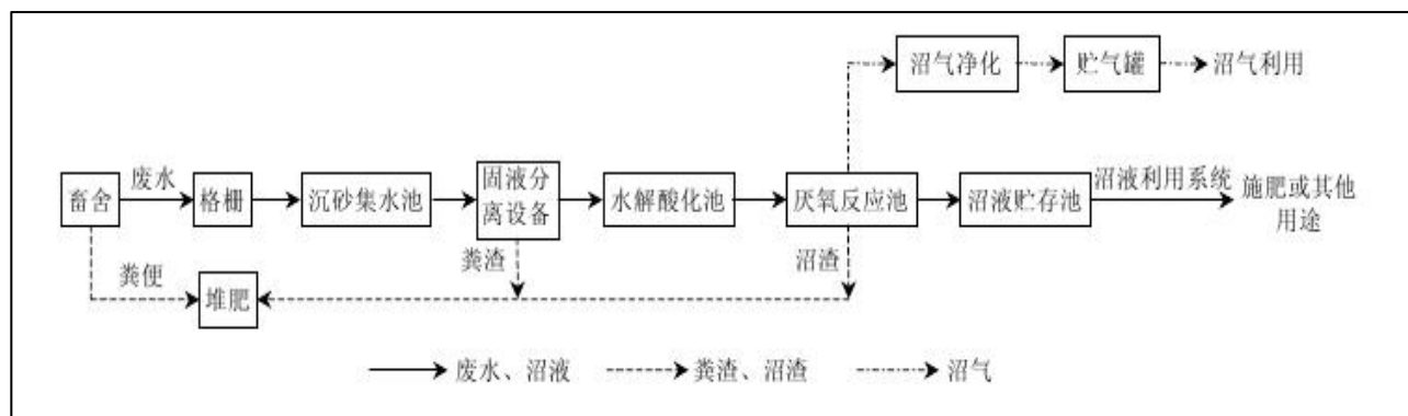
图 7-2-1 项目污水处理工艺流程图
