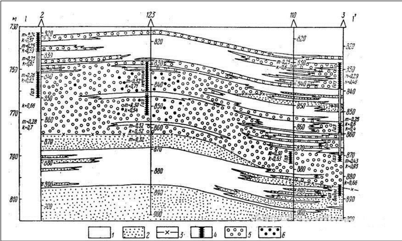
图 5-2-6 项目所在区域的地质剖面图
